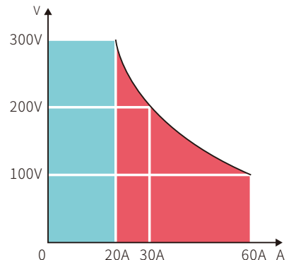
+ ITECH 操作范围 市面其他300V 产品操作范围
